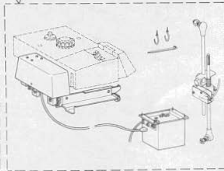
T013 Pedal switch type chain-off thread cutter ペダルスイッチ式糸切り装置
